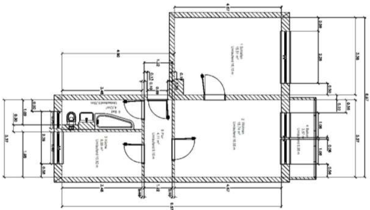
Grundriss
