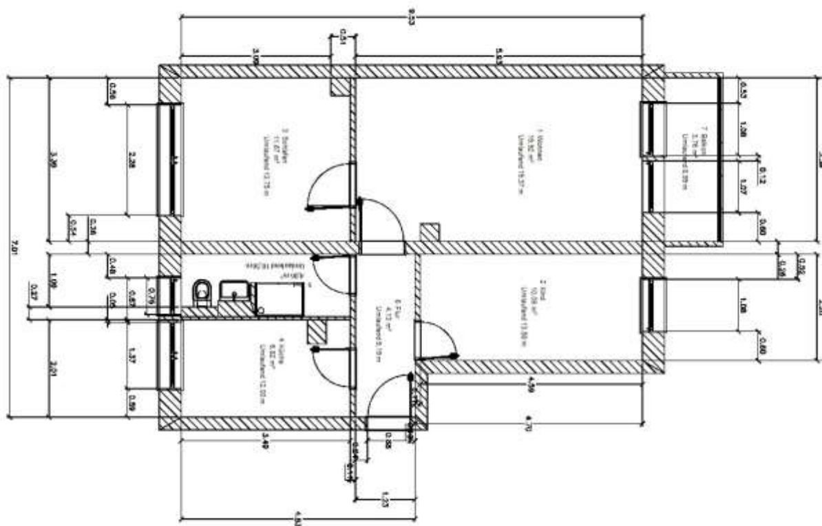
Grundriss
