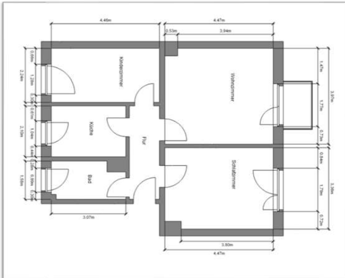
Grundriss
